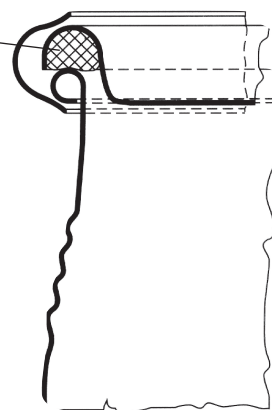
4. ábra A behúzott szájnyílás kialakítása
