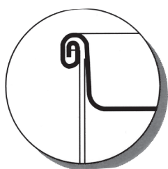
3. ábra Hétrétegű spirál korcolás
