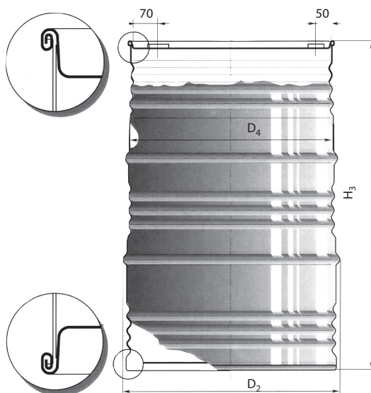
2. ábra 216,5 l-es sűrűn bordázott hordó
