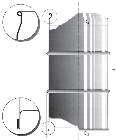
1. ábra 60 l-es behúzott szájnnyílású tonner
