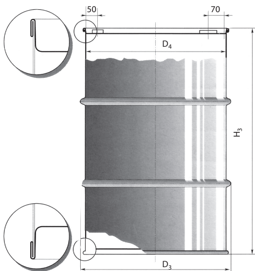
1. ábra 120–60–30 l-es hordó
