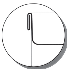
2. ábra Ötrétegű, lapos korcolás
