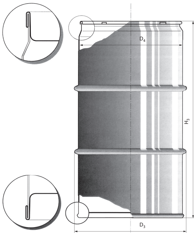
1. ábra 60 l-es hordó ODD tetővel
