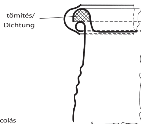
5. ábra A behúzott szájnnyílás kialakítása
