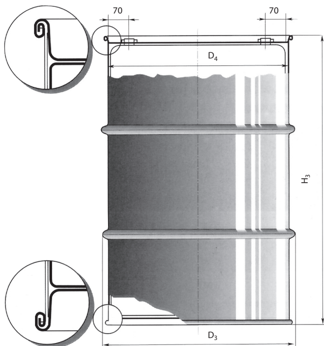
1. ábra 200–60 l-es polietilén-betétes hordó
