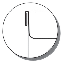
2. ábra Ötrétegű, lapos korcolás
