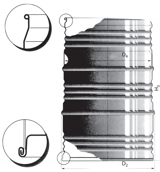
2. ábra 120 l-es sűrűn bordázott palástú tonner
