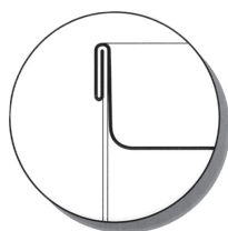
3. ábra Ötrétegű, lapos korcolás
