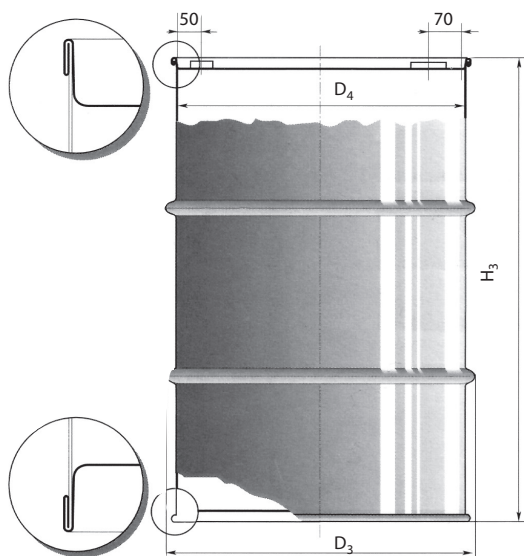
1. ábra 216,5 l-es hordó
