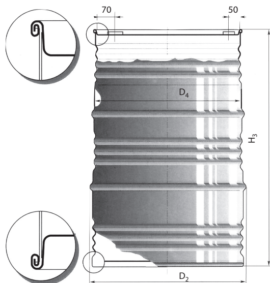
2. ábra 120 l-es sűrűnbordázott palástú hordó
