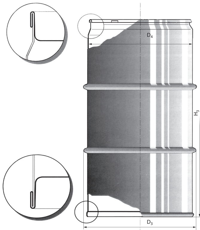
1. ábra 30 l-es hordó ODD tetővel
