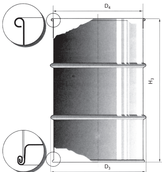
1. ábra 216,5–213 l-es paláستtal párhuzamos szájnyílású tonner
