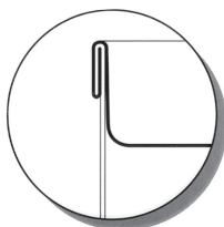
3. ábra Ötrétegű, lapos korcolás
