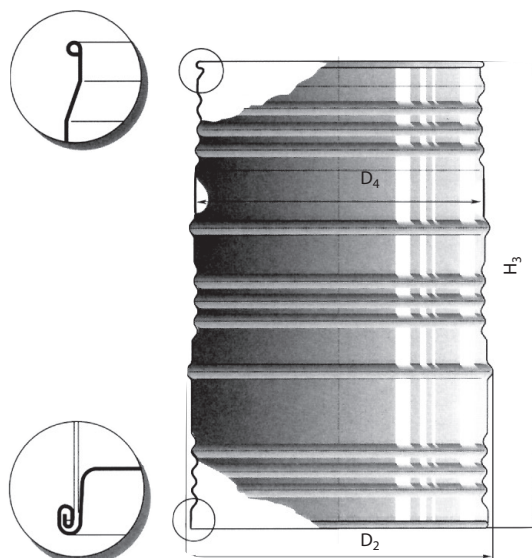
2. ábra 216,5–213 l-es sűrűn bordázott palástú, behúzott szájnyílású tonner
